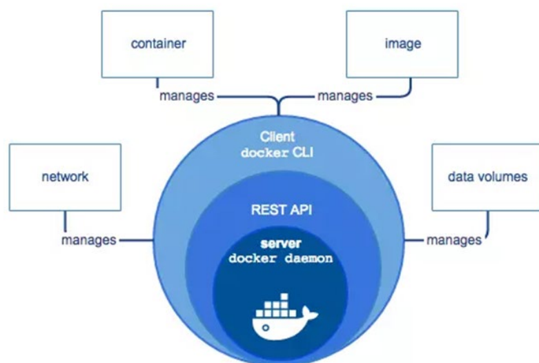
รูป 2.4 สถาปัตยกรรมของ Docker Engine
