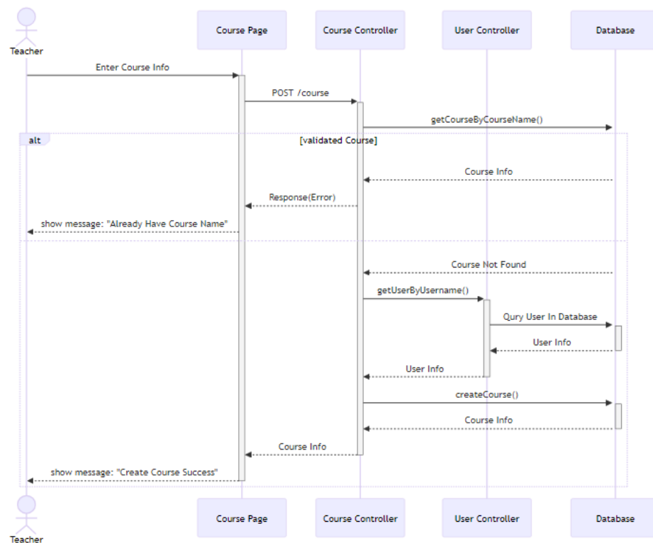
รูป 3.9 การทำงานของขั้นตอนการสร้างคอร์สเรียน
