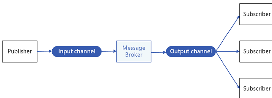
รูป 2.11 การส่ง (publisher) และ การรับ (Subscriber)
