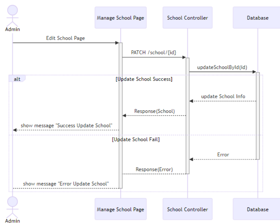
รูป 3.7 การทำงานของขั้นตอนแก้ไขสิทธิ์ของโรงเรียนโดยผู้ดูแลระบบ
