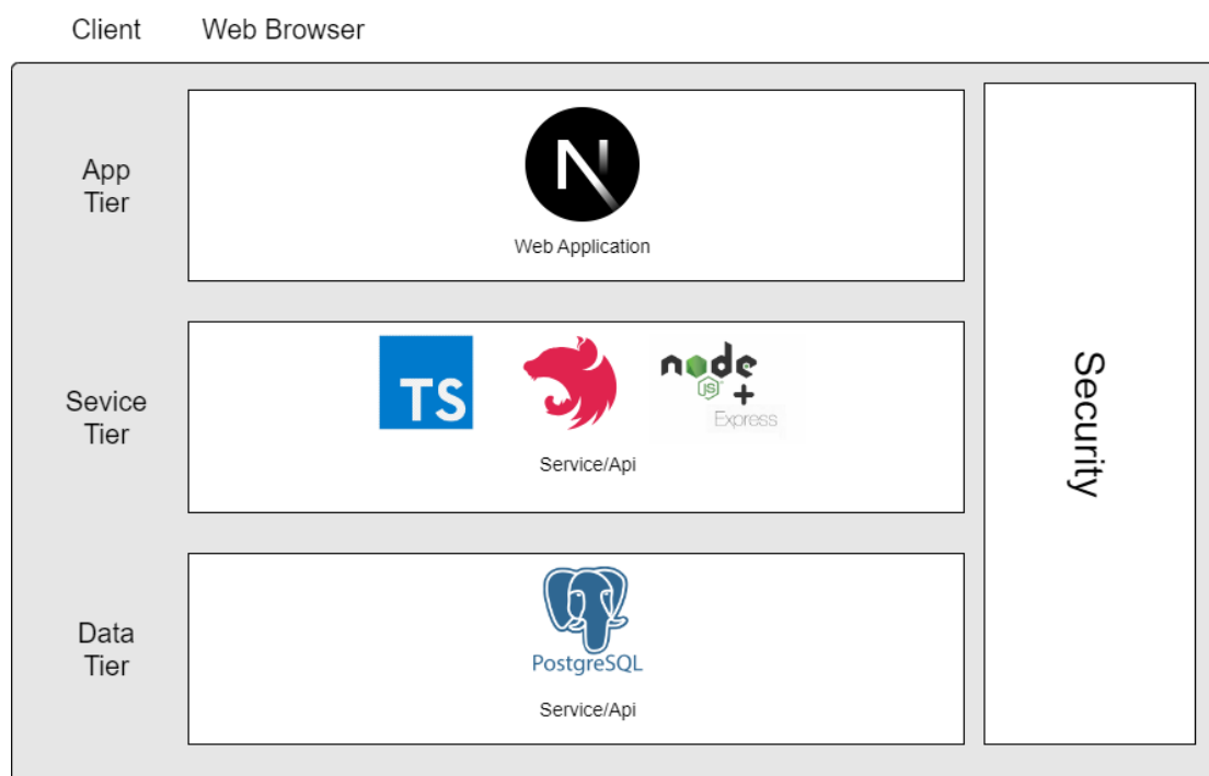
รูป 3.1 Three-Tier Architecture ของระบบแพลตฟอร์มเว็บแอปพลิเคชัน สำหรับเรียนรู้การพัฒนาการเขียนโปรแกรมในห้องเรียน
