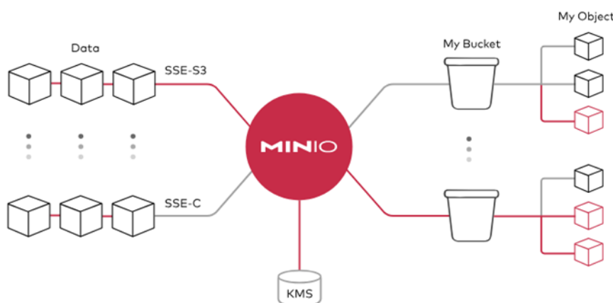
รูป 2.7 ภาพรวม MinIO
