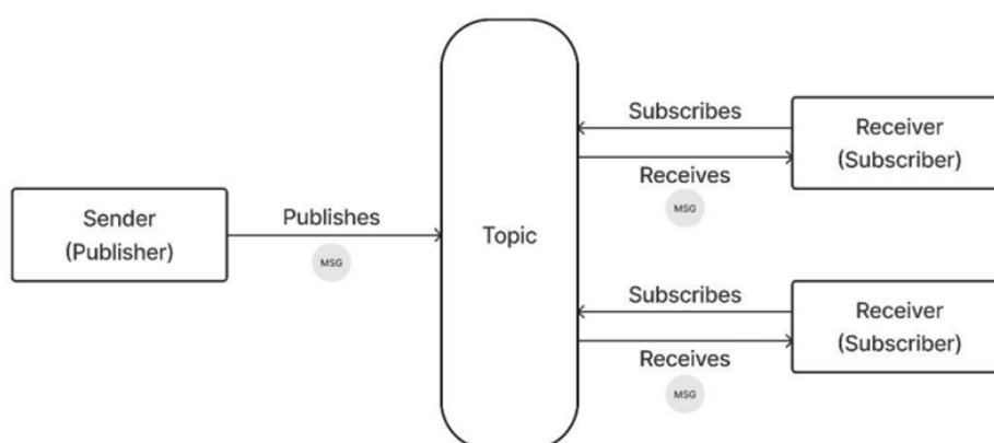
รูป 2.12 ภาพรวม Redis Pub/Sub
