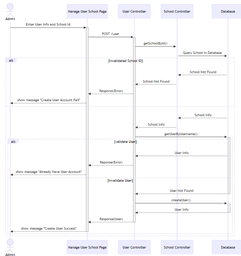
รูป 3.8 การสร้างบัญชีผู้ใช้งานโดยผู้ดูแลระบบ
