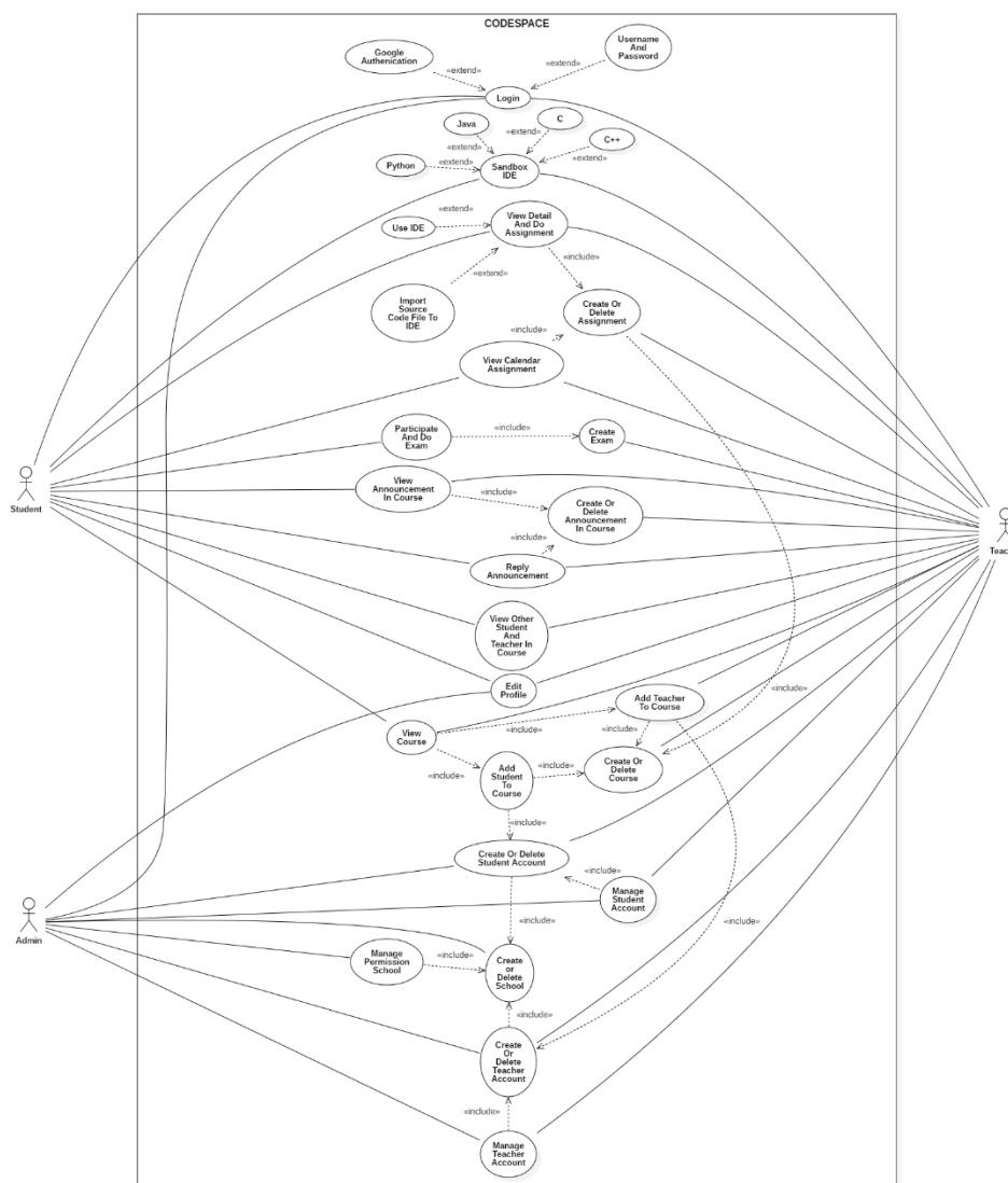
รูป 3.3 Use Case Diagram ของระบบแพลตฟอร์มเว็บแอปพลิเคชัน สำหรับการเรียนรู้การพัฒนาโปรแกรมในห้องเรียน
