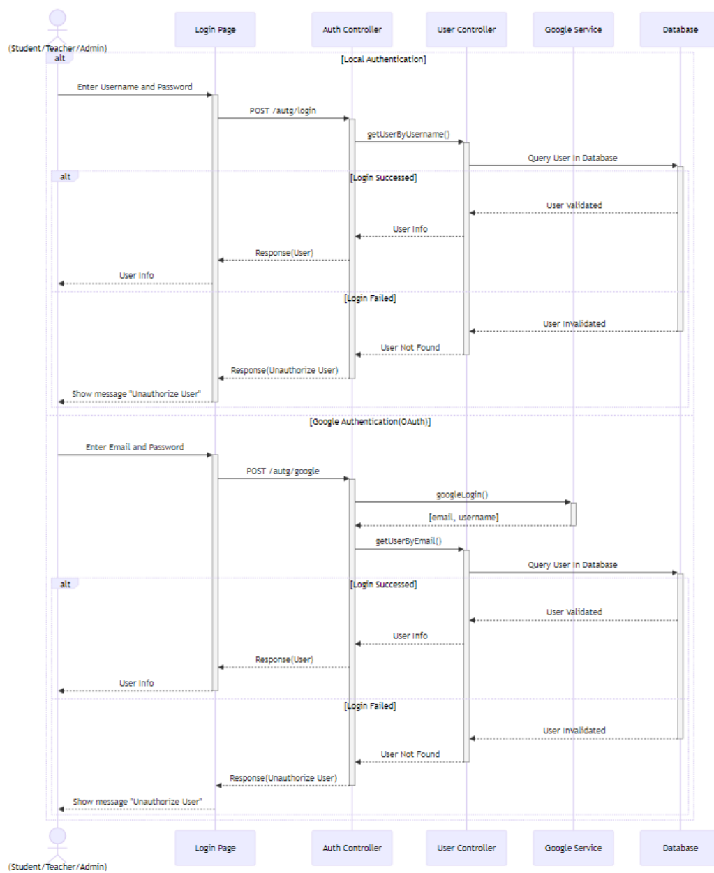
รูป 3.5 การทำงานของขั้นตอนการเข้าสู่ระบบ
