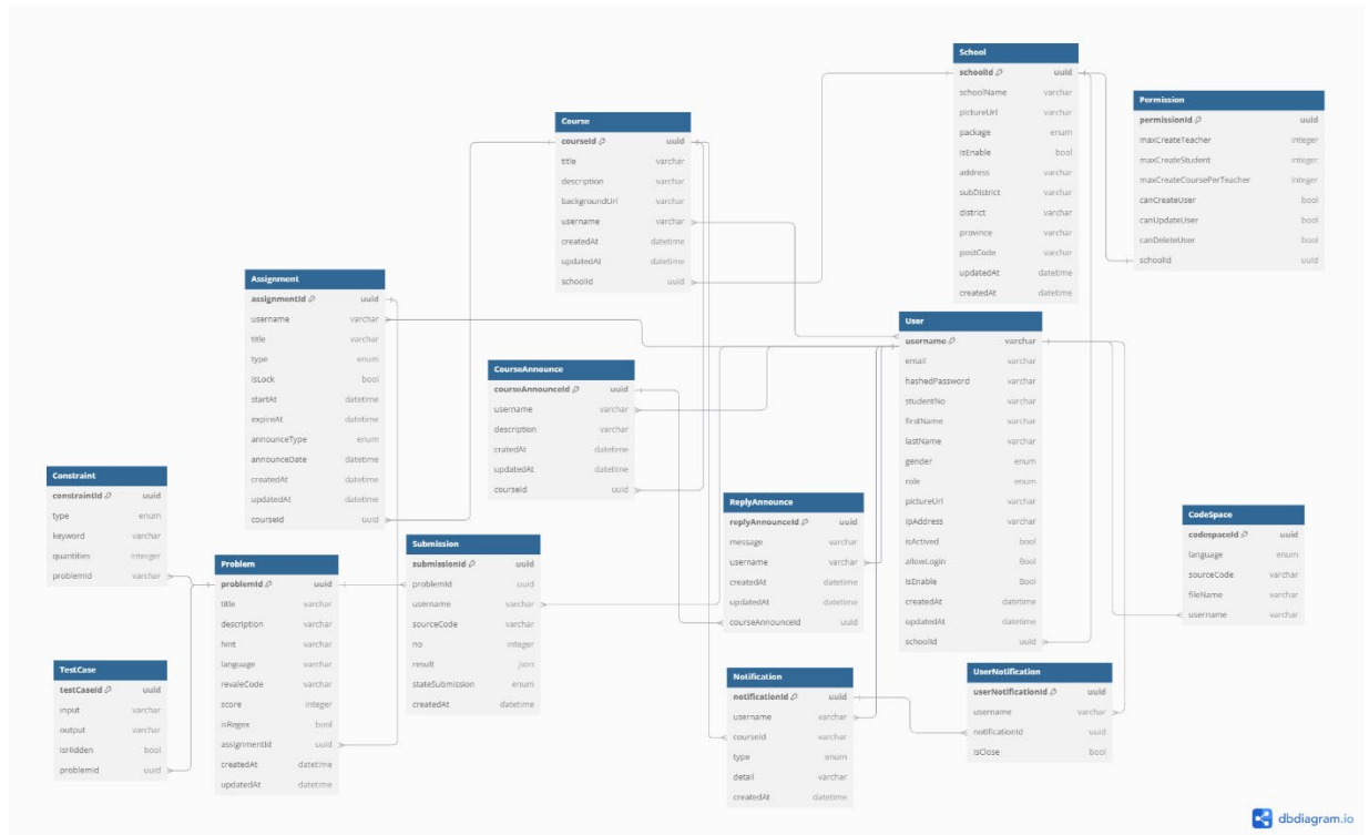
รูป 3.4 Entity Relationship Diagram ของระบบ
