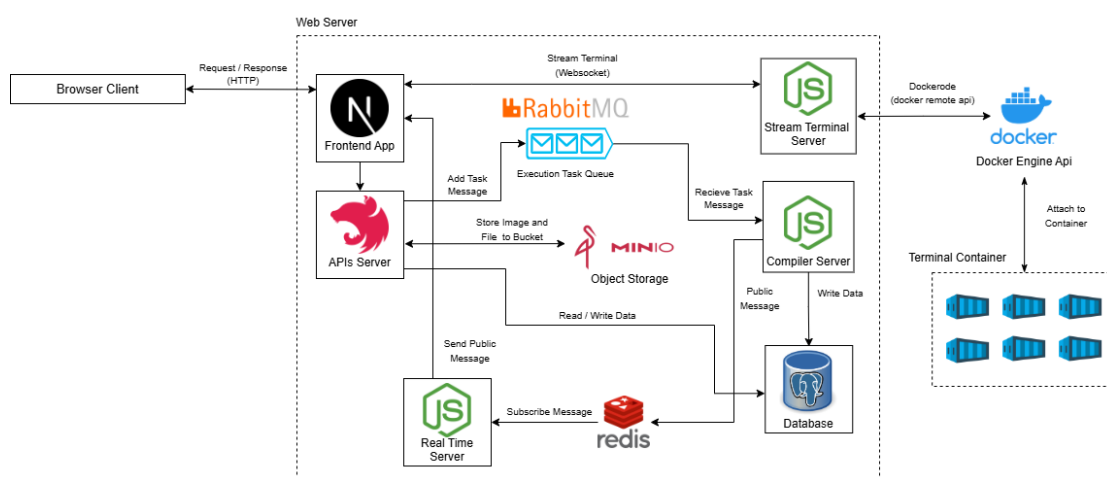
รูป 3.2 ส่วนประกอบของระบบของระบบแพลตฟอร์มเว็บแอปพลิเคชัน สำหรับเรียนรู้การพัฒนาการเขียนโปรแกรมในห้องเรียน
