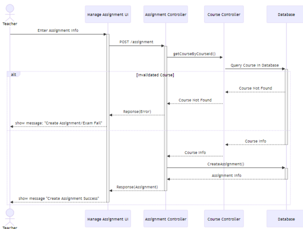
รูป 3.11 การทำงานของขั้นตอนการสร้างการบ้านหรือข้อสอบ
