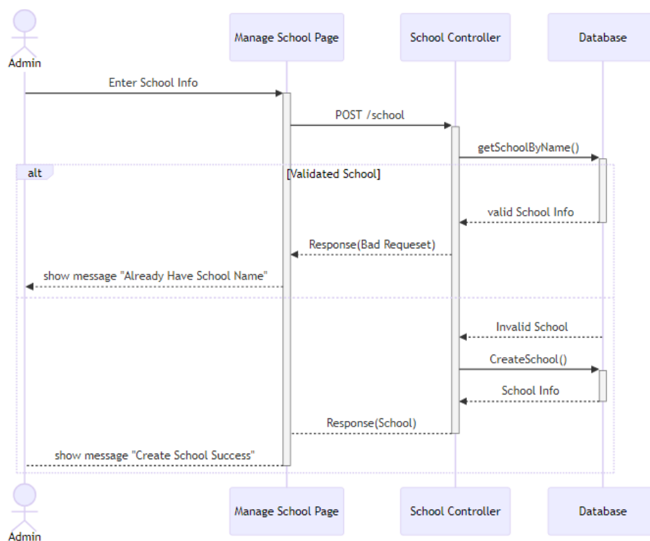
รูป 3.6 การสร้างข้อมูลโรงเรียน / สถาบัน โดยผู้ดูแลระบบ
