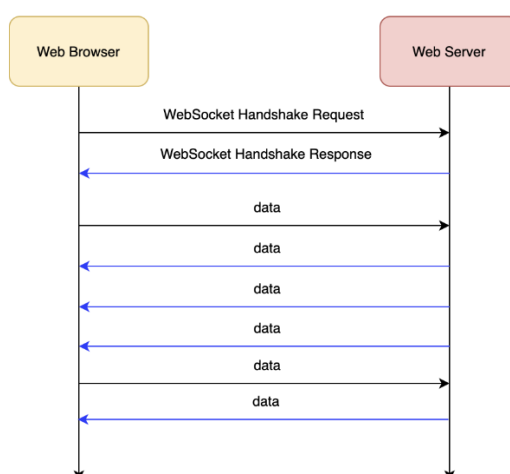
รูป 2.3 แผนภาพการติดต่อสื่อสารของ WebSocket Protocol
