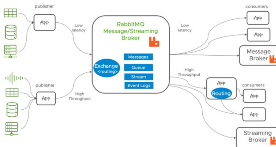
รูป 2.8 การทำงาน RabbitMQ
